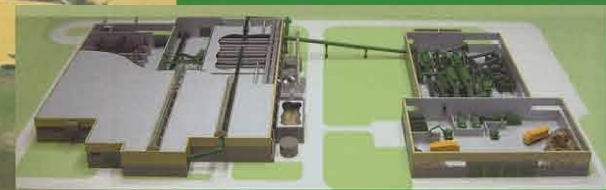
Modell der geplanten Mechanisch-Biologischen Abfallbehandlungsanlage
